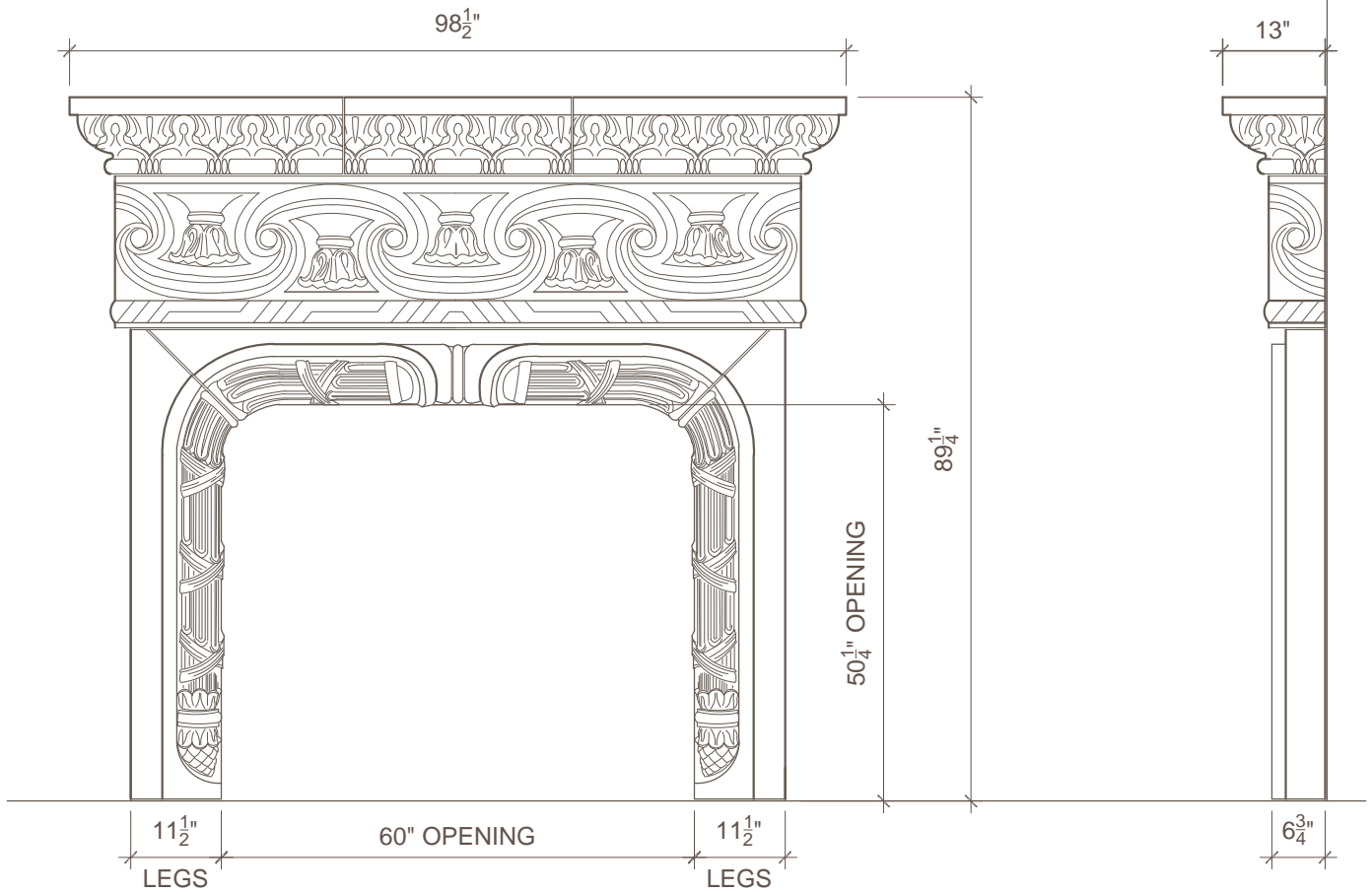
1 FRONT SCALE: 1/2" = 1'-0"
